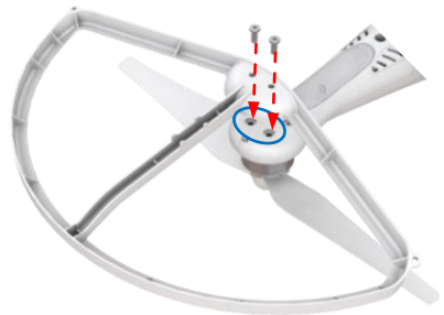
Fig.2 Prop Guard Attachment/图 2 安装桨保护器
